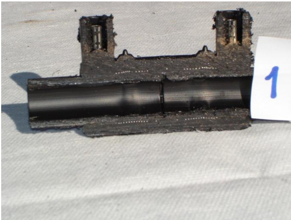
Slika 4.1. Presjek cijevi i elektrospojnice kod uzorka br.1 [13]
