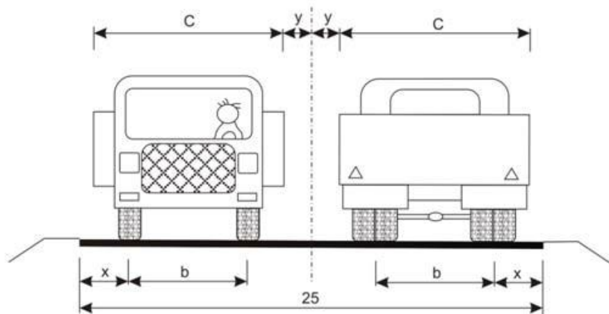
Slika 3.5: Širina prometnog traka (Rezo, 2016.)
