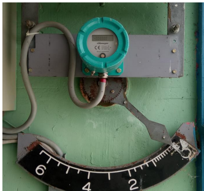
Slika 2.11. Rittmayer-ov davač položaja
