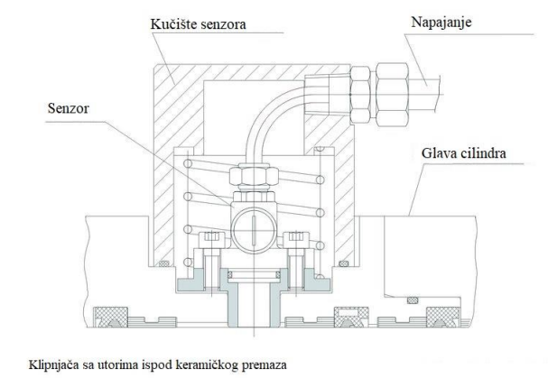
Slika 5.9. Prikaz dijelova senzora [7]
