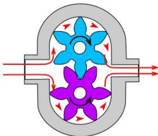
Slika 2.3. Zupčasta pumpa s vanjskim ozubljenjem [2]
