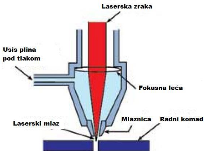
Slika 5.1 Princip laserskog rezanja [14]
