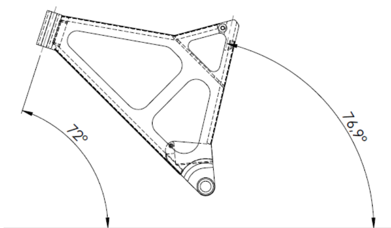
Slika 6.2 Prikaz kutova cijevi volana i cijevi sjedala
