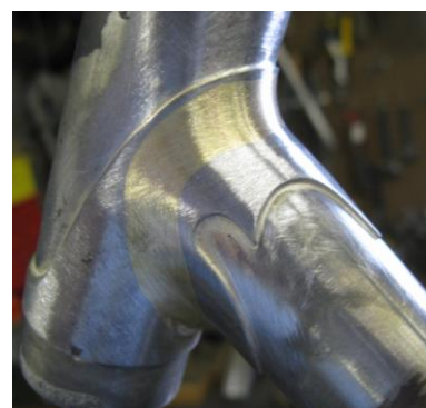
Slika 3.3 Spoj cijevi spojnom čahurom i tvrdim lemljenjem [7]
