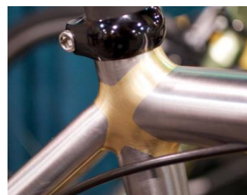
Slika 3.6 Spoj cijevi tvrdim lemljenjem [6]
