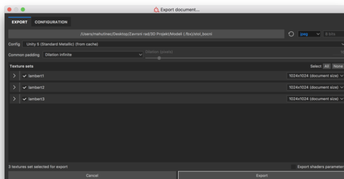
Slika 4.4. Exporting Textures
