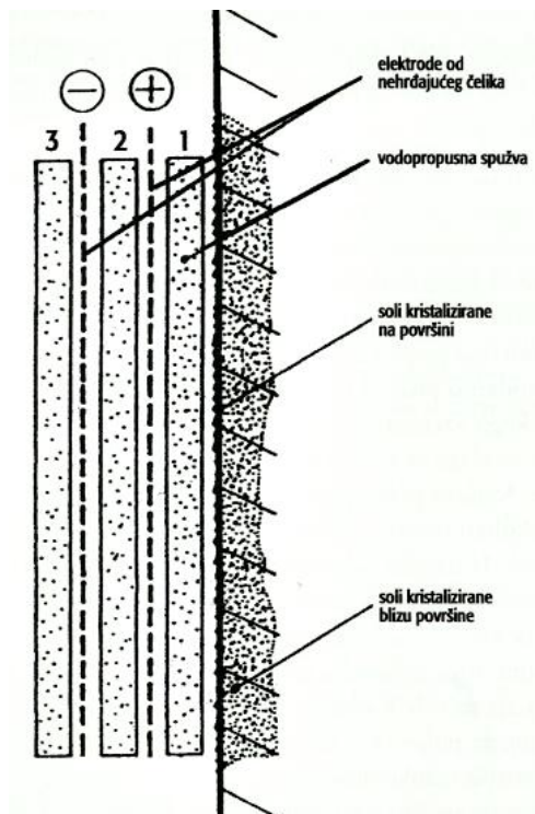
Slika 38. Prikaz elektrosendviča
