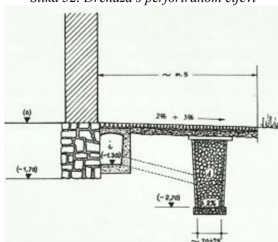
Slika 33. Zračni kanal sa odvodnjom prema bunaru
