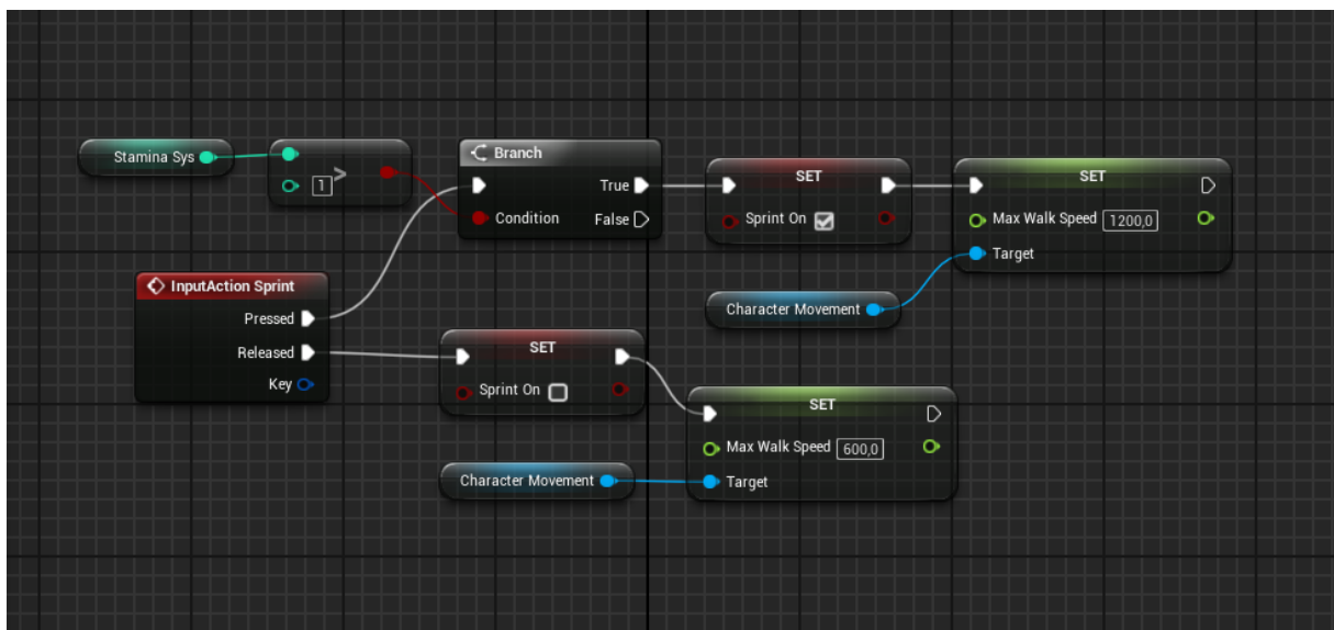
Slika 3.1: Primjer "Sprint" blueprintsa igre
