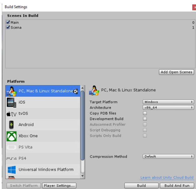
Slika 6.69. Build Settings
