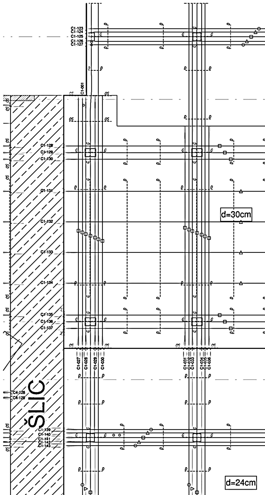
Slika 3.3 Nacrt vođenja kabela na promatranom segmentu
