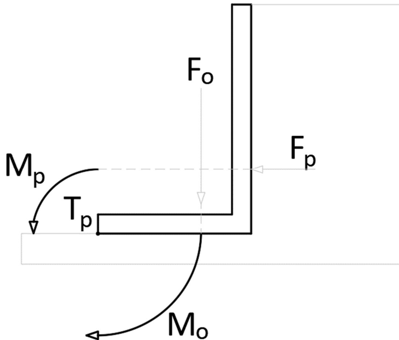
Slika 2.4.2. Prevrtanje
