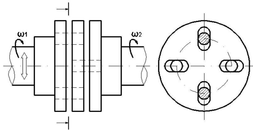
Slika 2.10 Oldhamova spojka s valčićima
