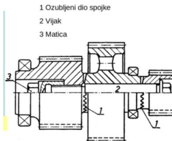
Slika 2. 6 Hirthova spojka
