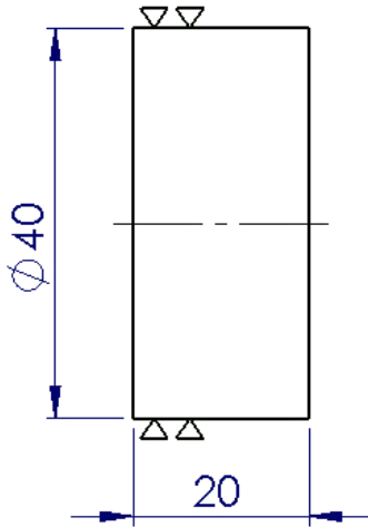
Slika 3. 6 Piljenje
