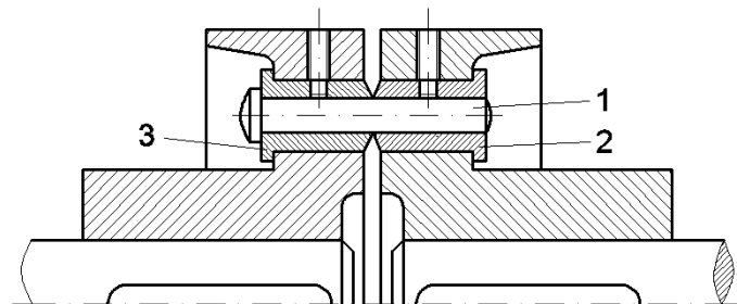
Slika 2. 19 Sigurnosna spojka
