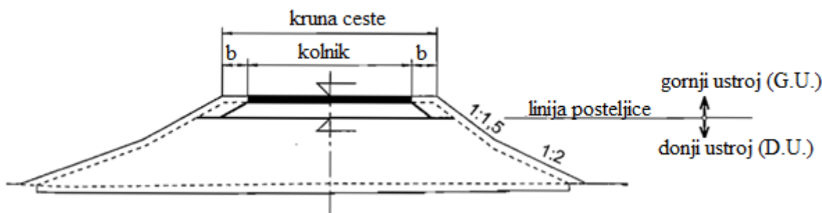
Slika 2.1. Trup ceste na nasipu
