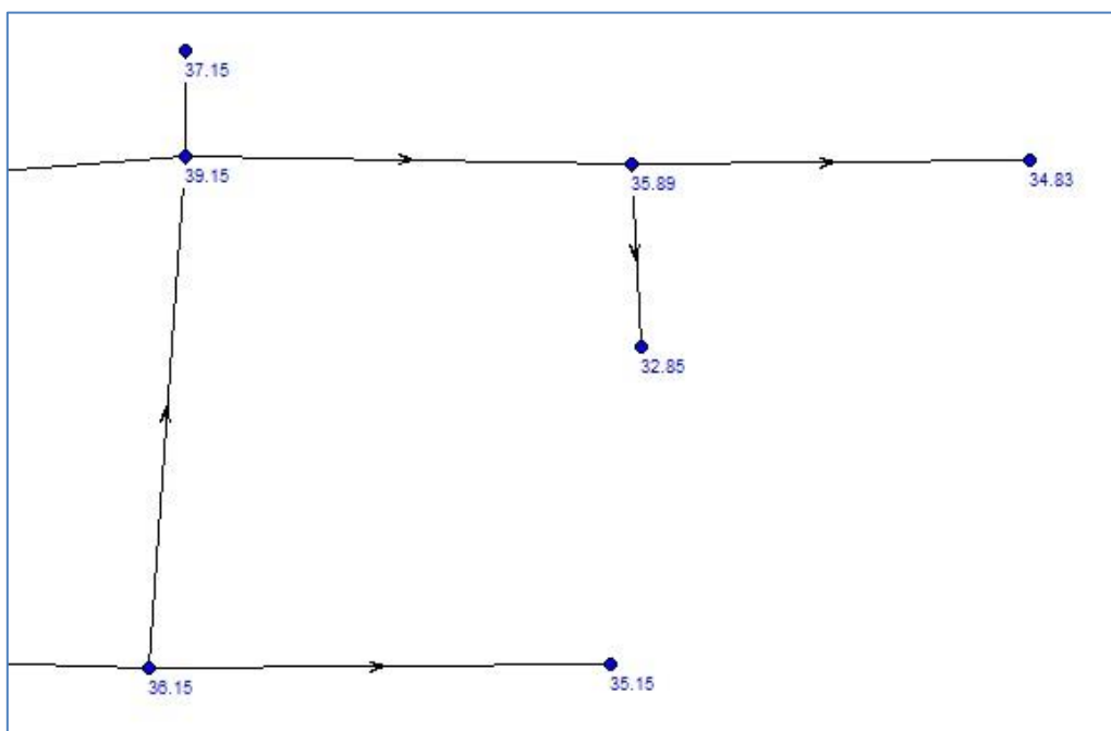
Slika 4.7 Odabrani dio cjevovoda promjera 50 [mm]
