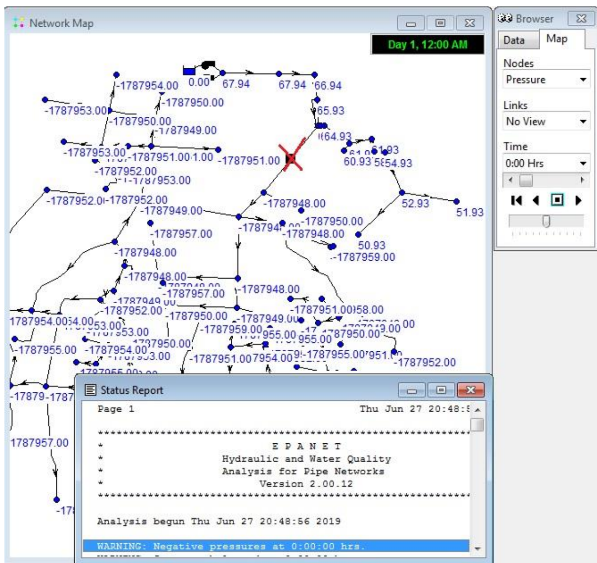
Slika 4.3 Granata mreža nakon puknuća cijevi
