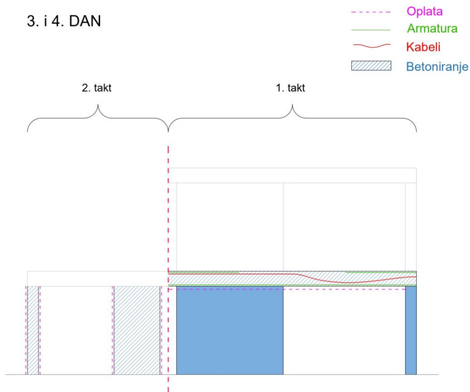
Crtež 5.4 Prikaz sheme izvođenja radova 3. i 4. dan
