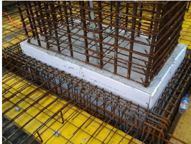
Slika 3.5 Prikaz dilatiranja stupa
