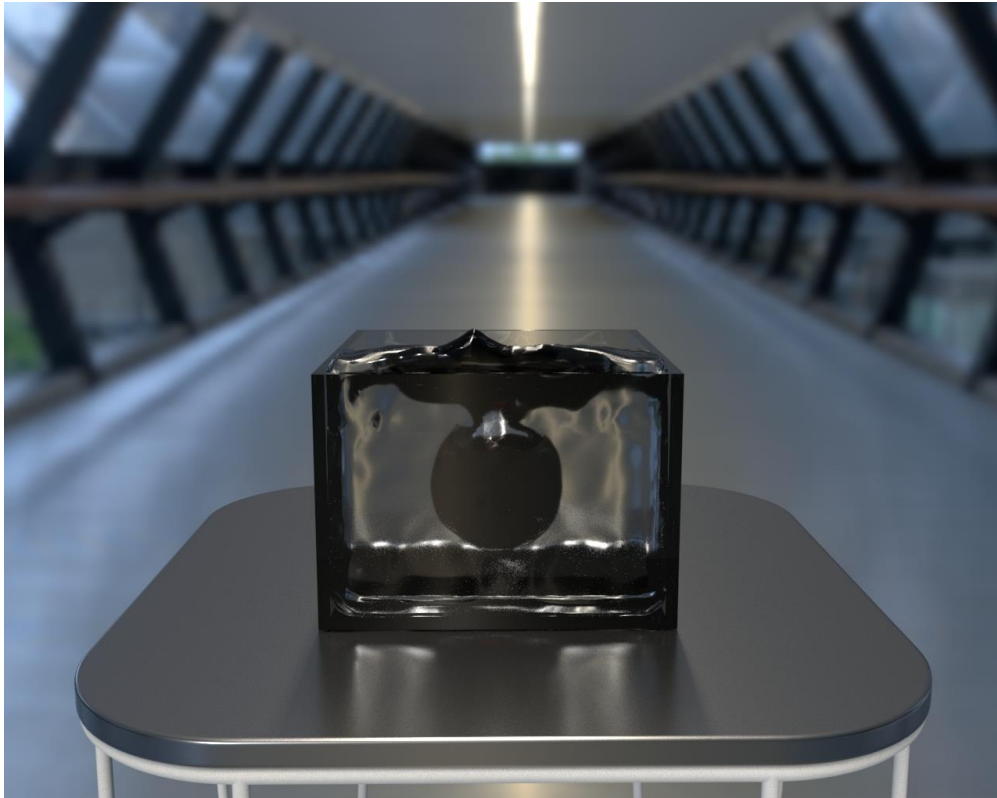
Slika 10.35 Bifrost render
