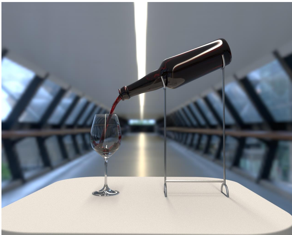
Slika 10.24 Bifrost render
