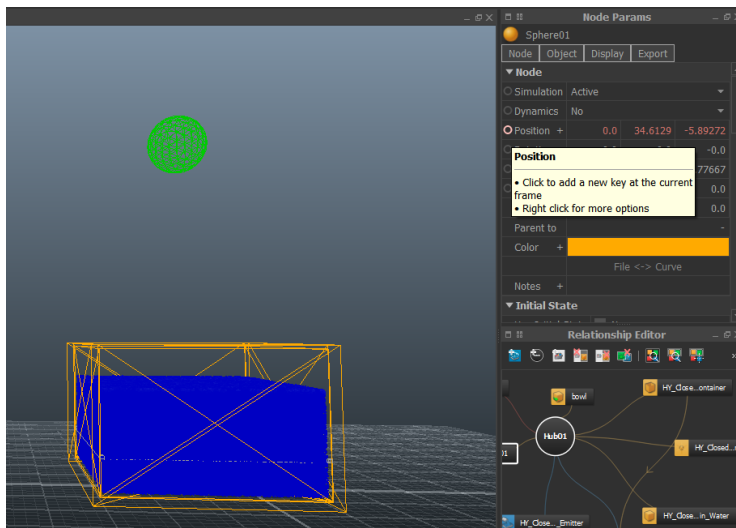
Slika 10.33 Animiranje kugle
