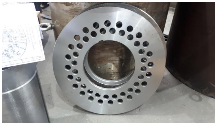
Slika 2.13 Tlačna ploča sa provrtima za hlađenje paketa
