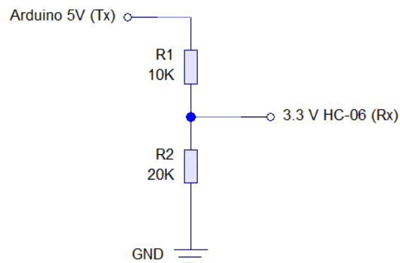
Slika 4-2. Naponski djelitelj
