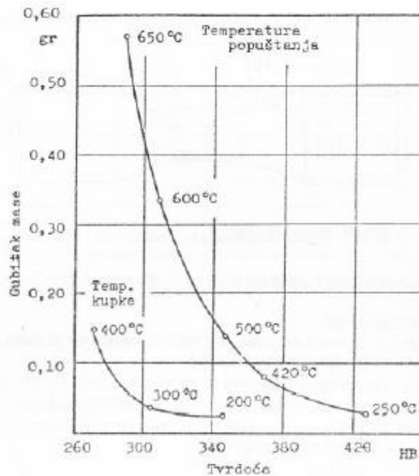
Slika 2.9: Usporedba trošenja kaljenog (i popuštenog) i izotermički poboljšanog sivog lijeva, [10]
