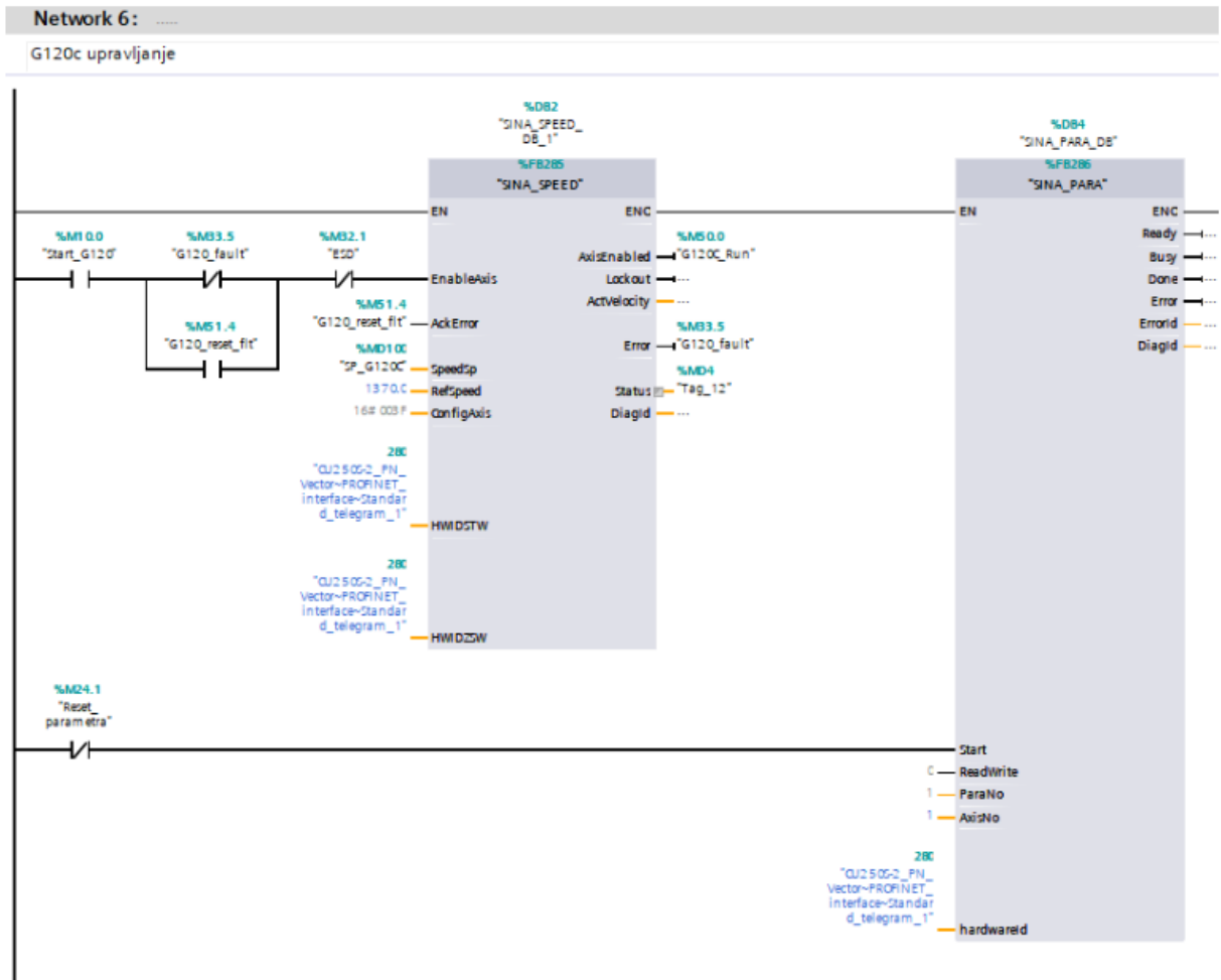
Slika 7.5 Sina_para i Sina_speed blokovi za G120C
