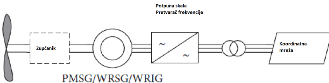
Slika 3.4. Model vjetroagregata sa sinkronim strojem s kliznim kolotima
