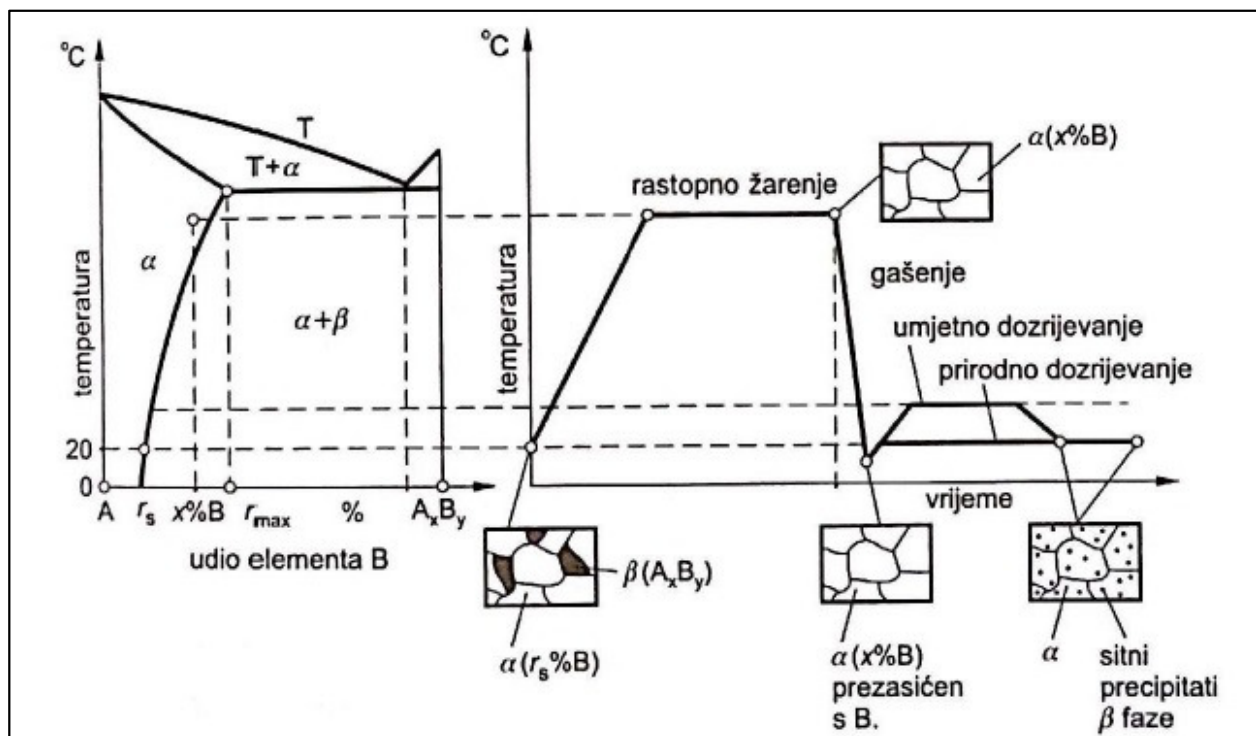
Slika 2.4 Dijagram stanja za precipitacijsko očvršnuće [11]
