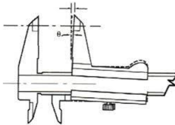
Slika 4.3. Nezadovoljavanje Abbe-ovog principa
