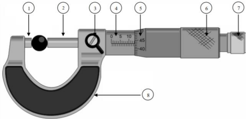
Slika 4.4. Dijelovi mikrometra
