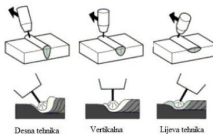
Slika 8.12 Vrste zavarivanja
