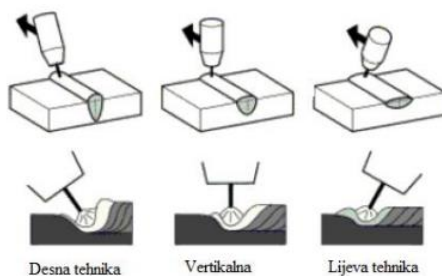
Slika 8.12 Vrste zavarivanja
