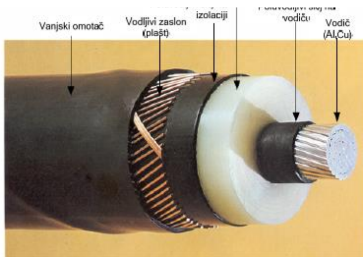
Slika 3.14 Jednožilni kabel
