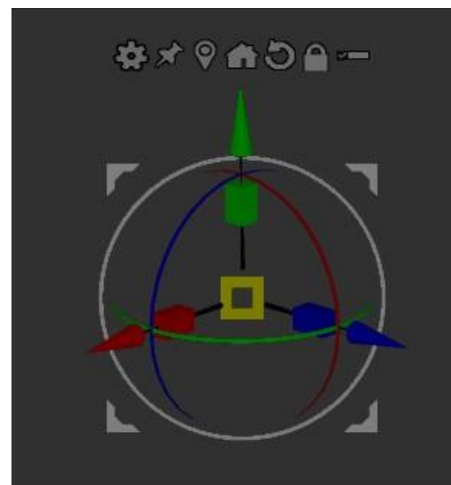
Slika 3.2.9. „Transpose“ alat
