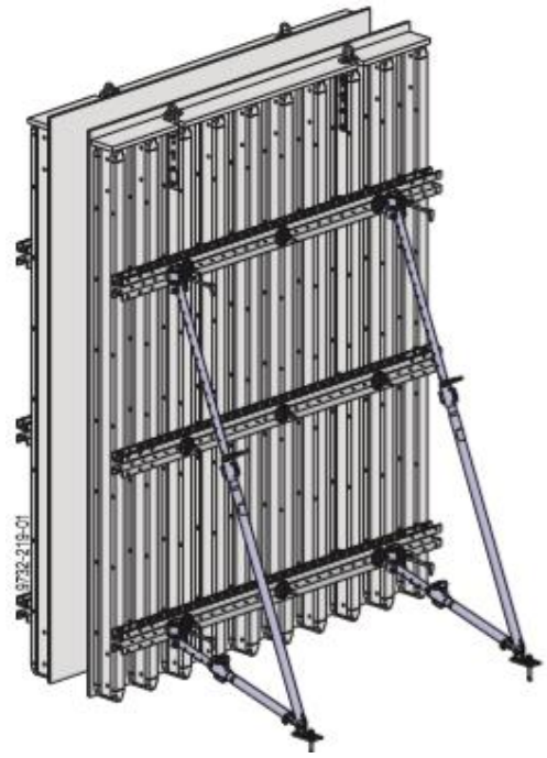
Slika 3.13. Skica kosnika
