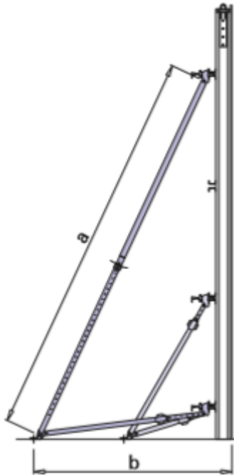
Slika 3.14. Kosnik 540
