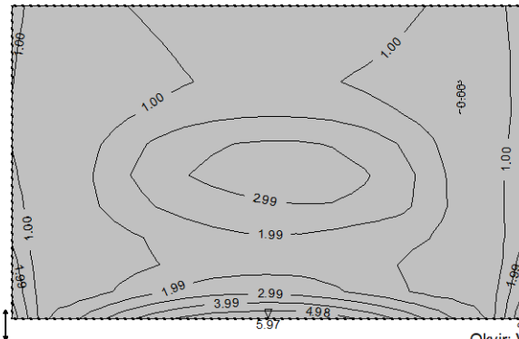
Okvir: V_3 Aa - d.zona - Pramac 2 - max Aa2,d= 5.97 cm²/m
