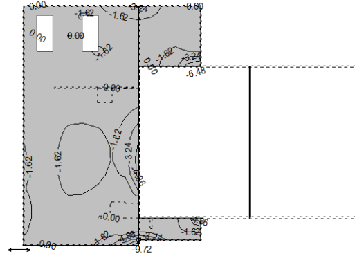
Okvir: V_2 Aa - g.zona - Pravac 1 - max Aa 1,g = -9.72 cm 2 /m
