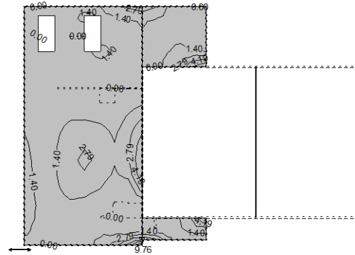
Okvir: V_2 Aa - d.zona - Pravac 1 - max Aa 1,d = 9.76 cm 2 /m
