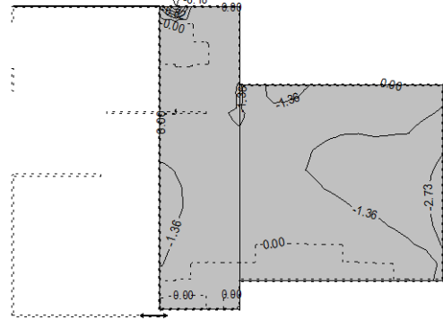
Okvir: V_5 Aa - g.zona - Pravac 1 - max Aa 1,g = -8.18 cm 2 /m
