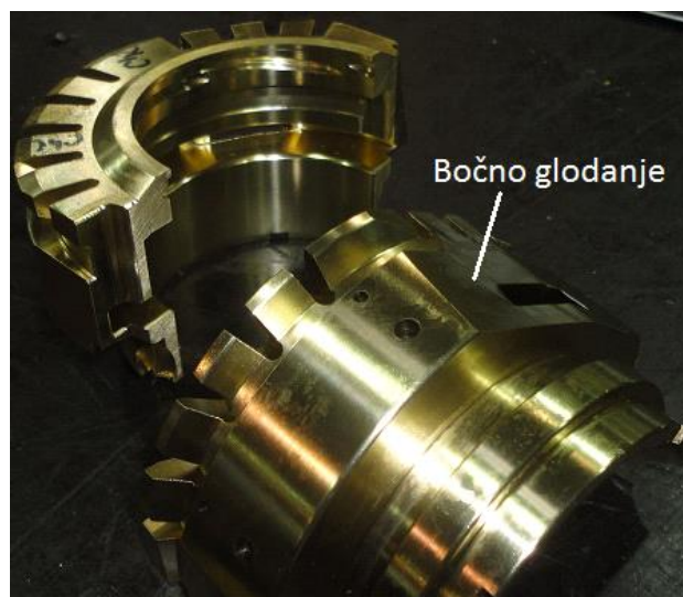
Slika 6.26. Bočno glodanje [15]
