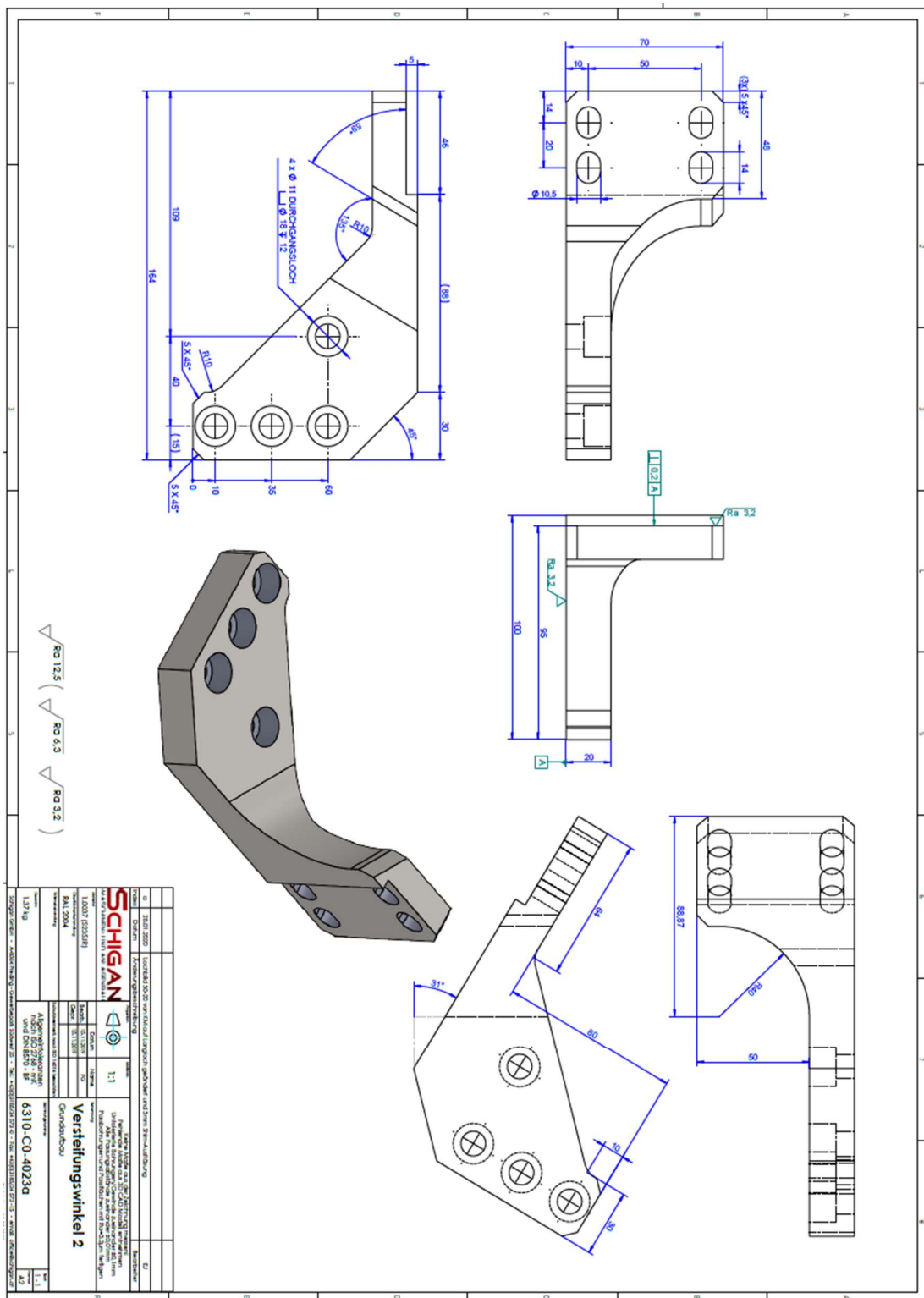
Slika 8. Strojni crtež za izradak
