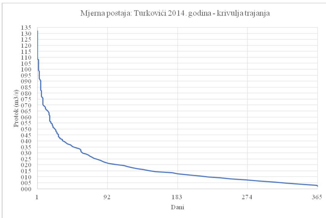
Prilog 11.4.6. Grafički prikaz krivulje trajanja protoka postaje Turkovići za 2014.god.
