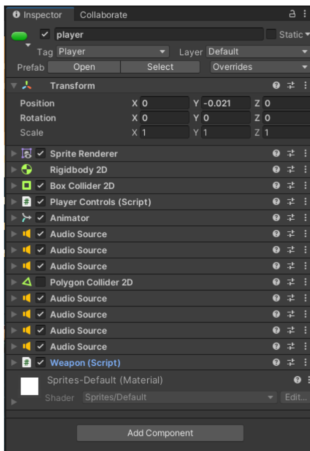
Slika 11: Prozor Inspektor
