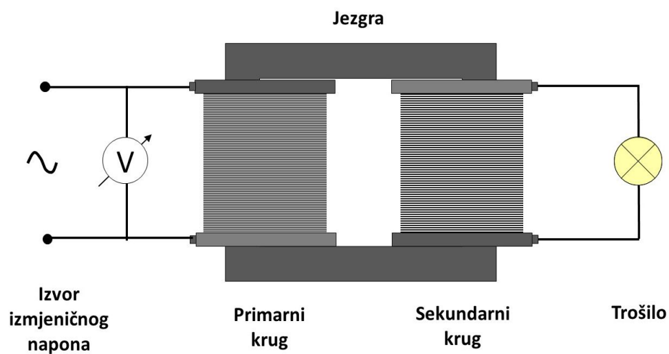
Slika 3.9. Transformator [17]
