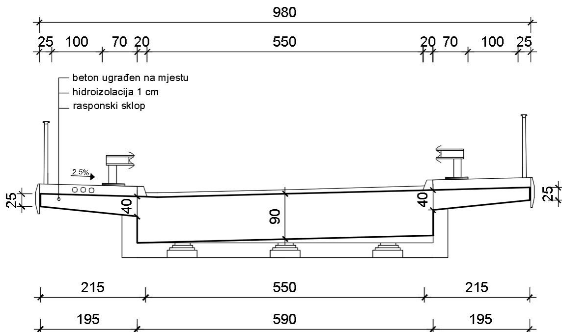
Slika 6.) Poprečni presjek i dimenzije za proračun u programu Tower
