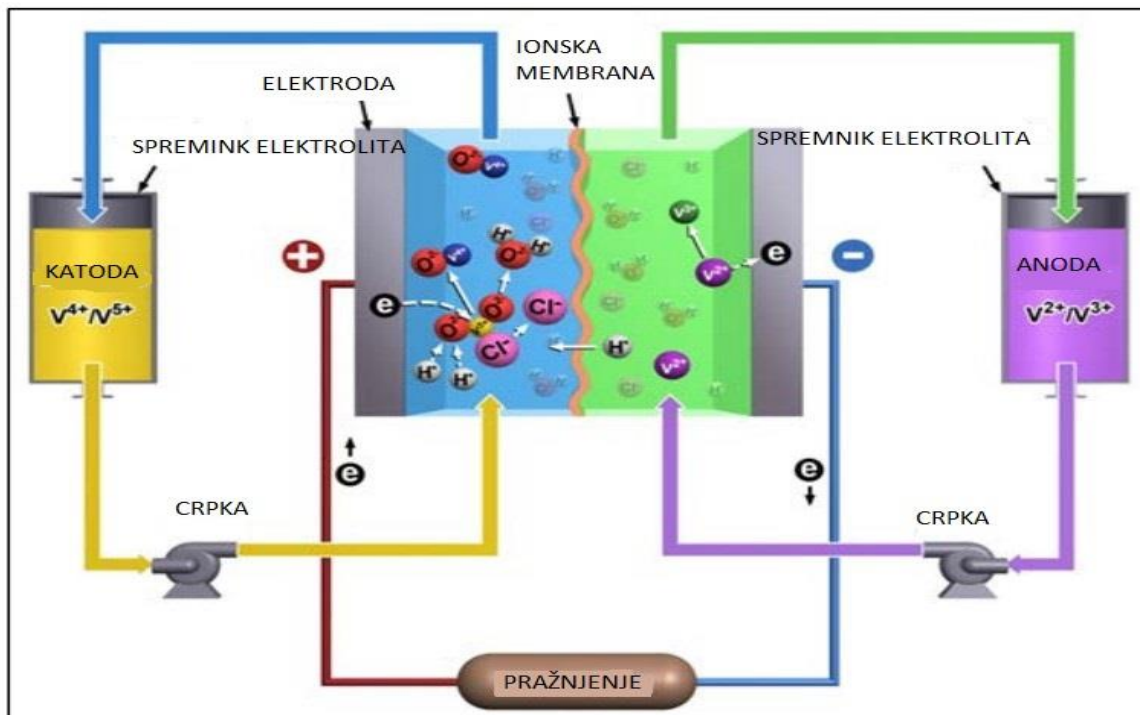
Slika 3.16 Princip rada VRB baterije [2]
