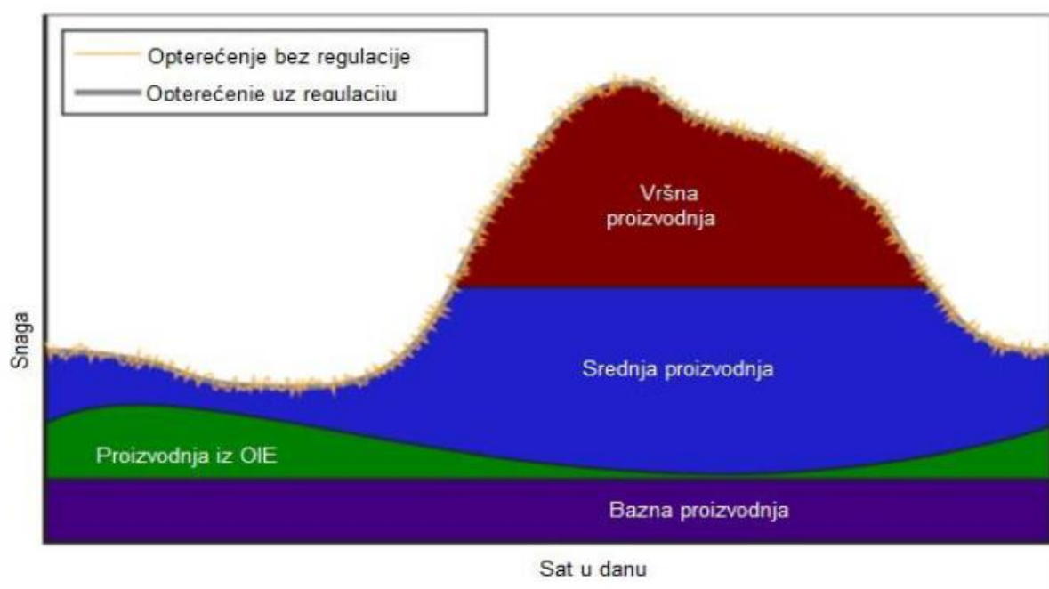
Slika 2.2 Prikaz opterećenja sa i bez regulacije [1]
