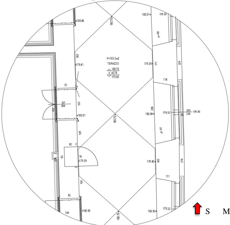
Slika 3.19 Analizirana prostorija hodnika na drugom katu (tlocrt)
