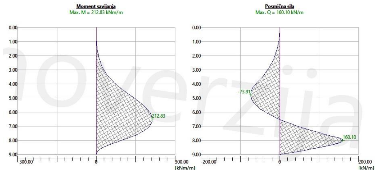
Slika 5.17. Unutrašnje sile.
