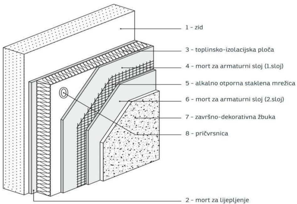
Slika 6.1. Primjer ETICS sustava
