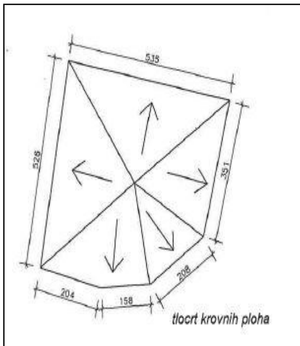
Slika 107. Tlocrt krovšta kule
