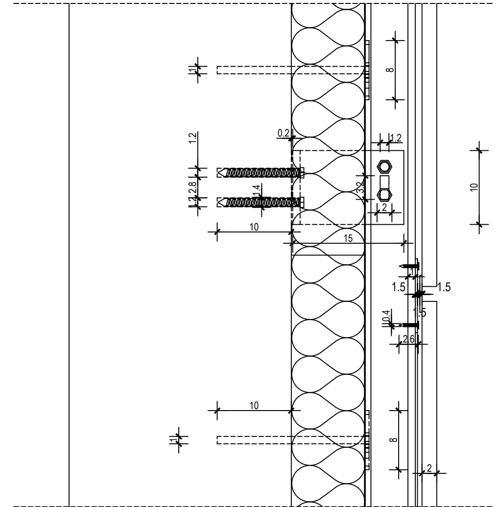
PRESJEK DETALJ 1:5
