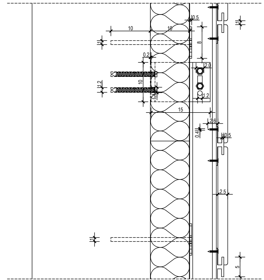
PRESJEK DETALJ 1:5
