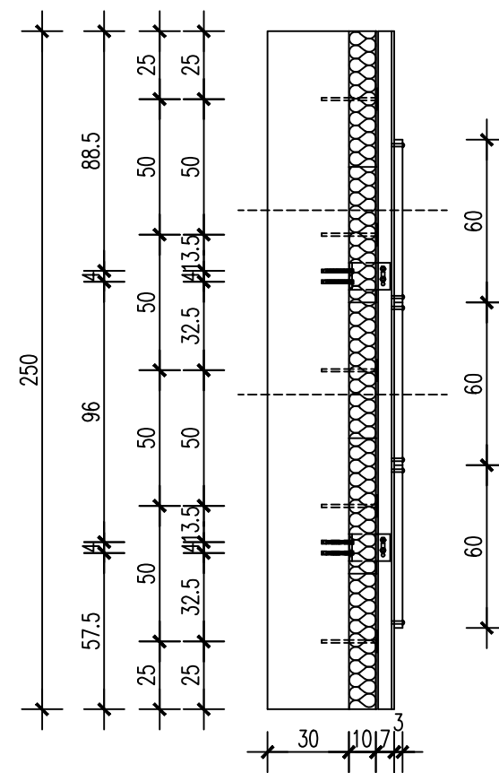
PRESJEK
