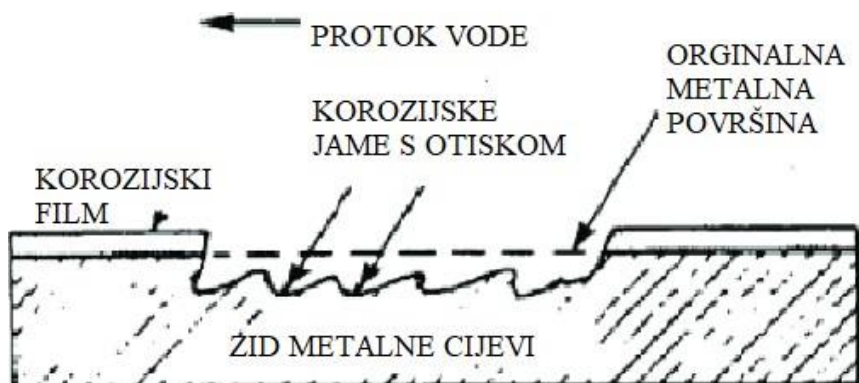
Slika 23. Erozija metala [15]
