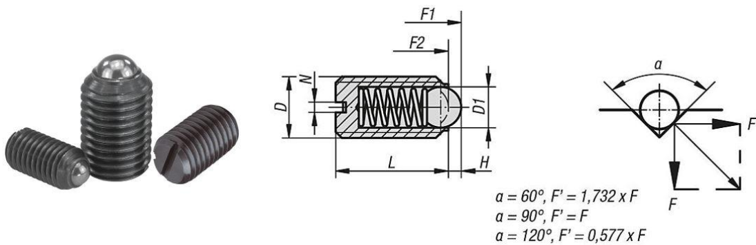
Slika 23. Prikaz odabranog vijka sa opružnim mehanizmom indeksiranja te njegove karakteristike [13]
