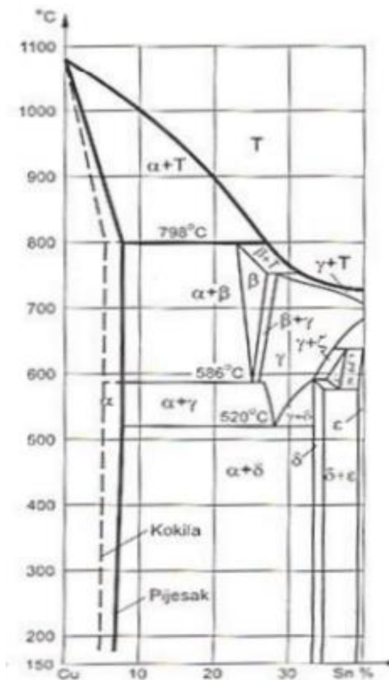
Slika 2.4 Dijagramski prikaz lijevanog stanja Cu – Sn [1].
