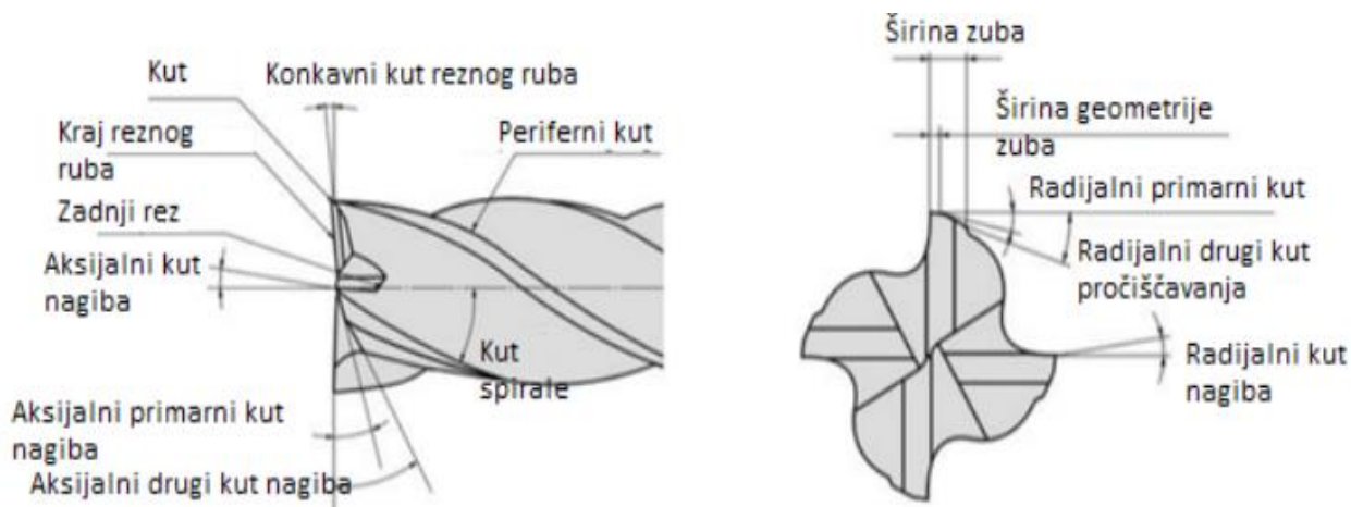
Slika 3.5 Geometrija alata [2]
