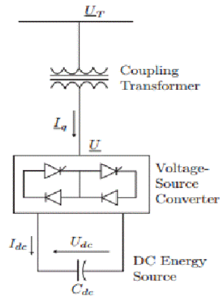
Slika 4.8 Shematski prikaz STATCOM-a [11]
