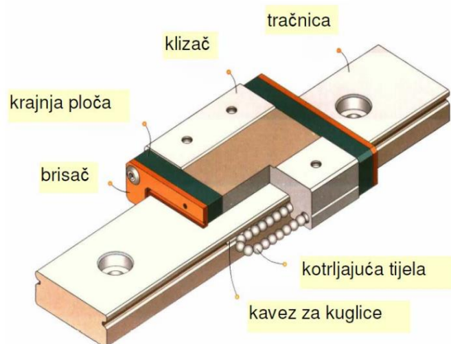
Slika 7 Kotrljajuća vodilica [11]
