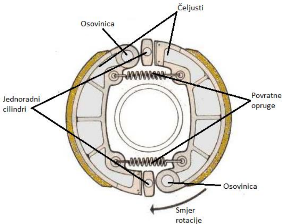
Slika 6. Duplex kočnica [4]
