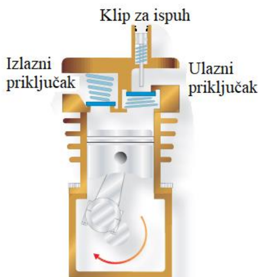
Slika 12. Kompresor [1]
