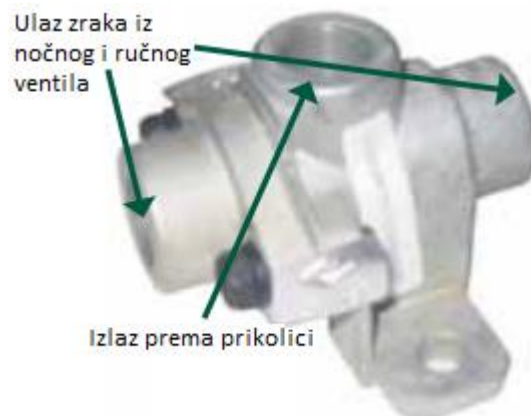
Slika 40. Dvosmjerni nepovratni ventil [1]
