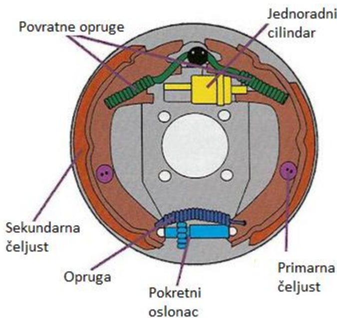
Slika 7. Duo servo kočnica [5]
