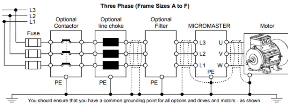
Slika 9. Dijagram spajanja pretvarača [7]
