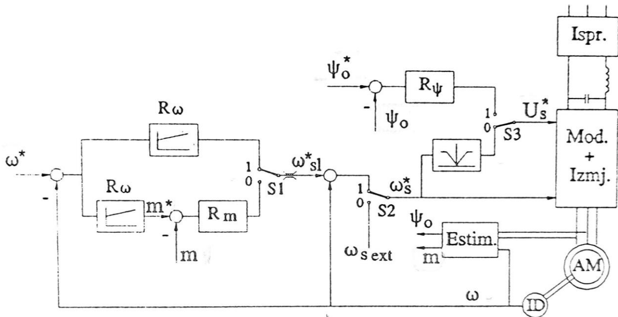
Slika 6. Skalarno upravljanje naponom statora [3]
