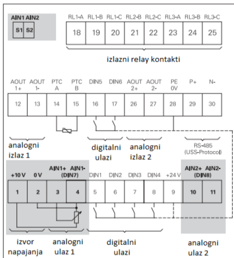
Slika 8. Ulazi i izlazi pretvarača [6]
