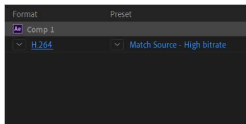
Slika 55 Metoda kompresije
