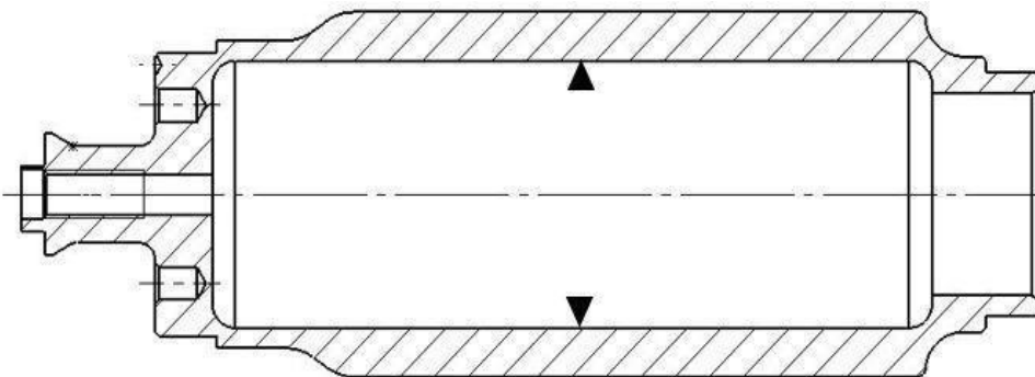
Slika 6.7 Operacija 30, zahvat 1
