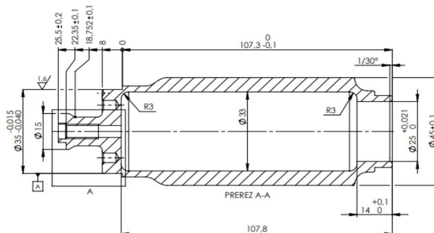
Slika 5.4 Konačne dimenzije proizvoda
