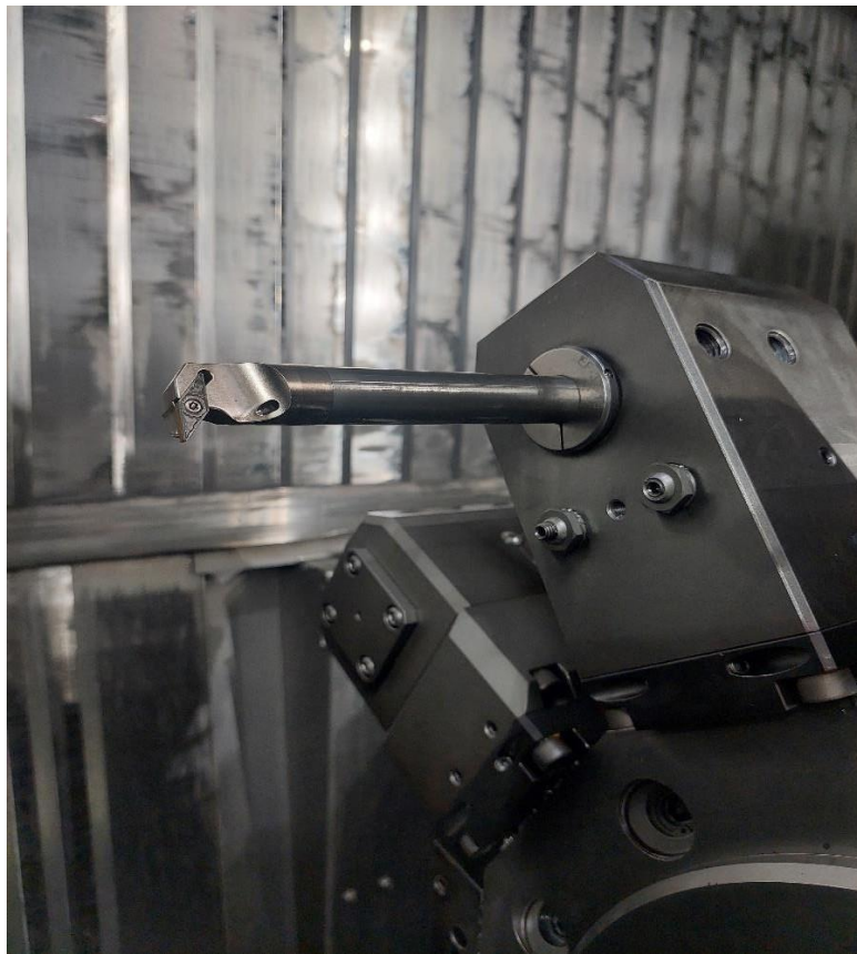
Slika 6.5 Držač „A12M-SDXCR 07-R“ i pločica „DCMT 07 02 08-UM 4425“
