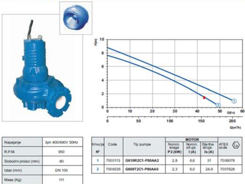
Slika 3.1. Odabrana crpka [17]
