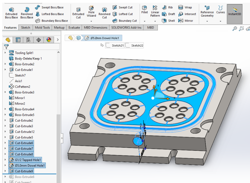
Slika 50 Oblikovanje sustava za odzračivanje
